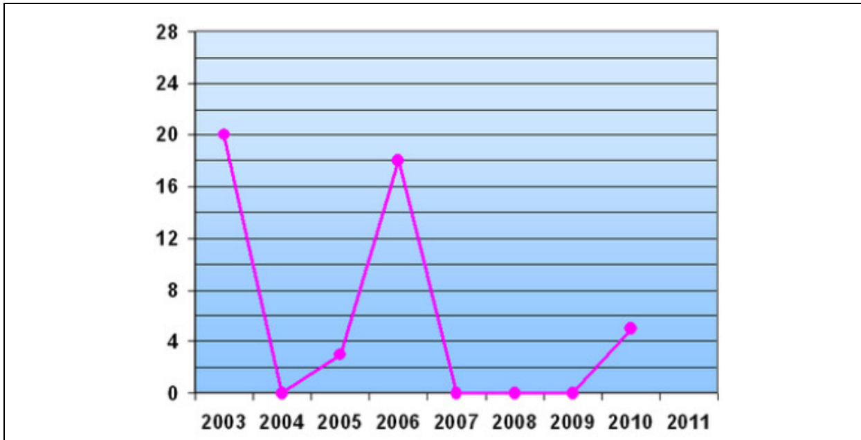
Abb. 65 Anzahl der Ozon-1h-Messwerte (Stundenmittelwerte) größer als 180 /g/m 3 pro Jahr im städtischen Hintergrund für Sachsen-Anhalt
