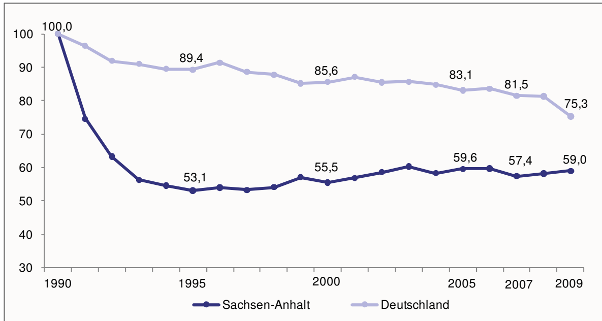
Abb. 44 Entwicklung der energie- und prozessbedingten CO 2 -Emissionen 1990 bis 2009 (1990 = 100)
